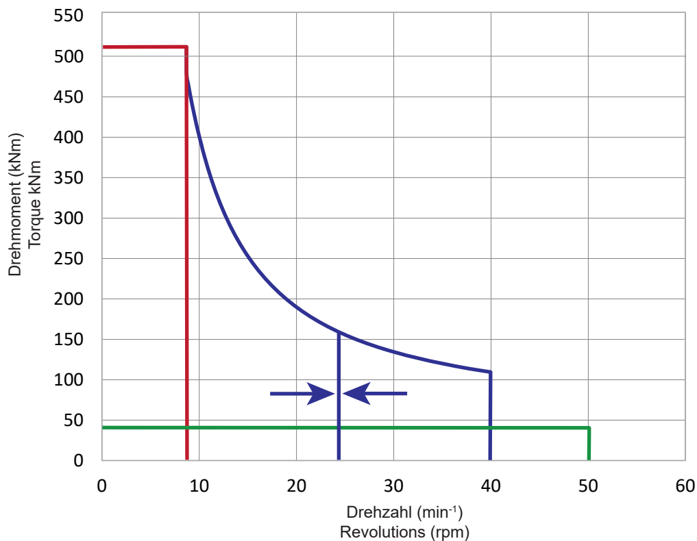
Kellybohrantrieb BT 500 / Rotary Head BT 500
