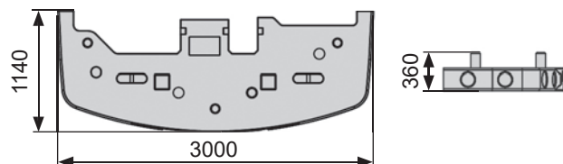
Konsole für Gegengewicht / Base plate for counterweight
